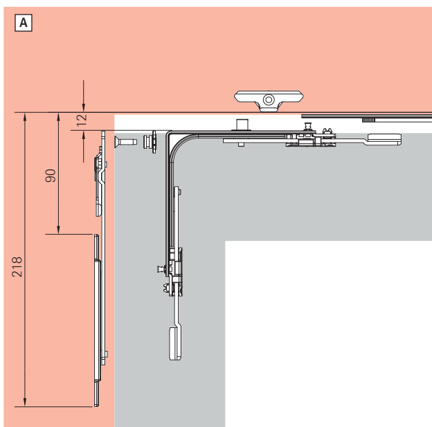
[А] Установка фрамужных ножниц сбоку
