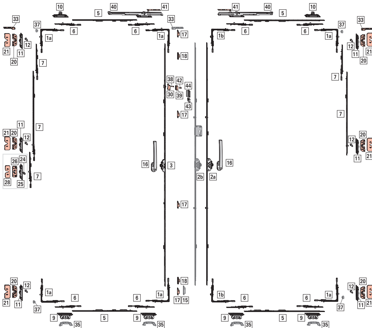
Илл. 3.3: на рис.: ПВХ; исполнение: активная створка DIN L запор DM 35, вторая открываемая створка DIN R запор DM 25; ШСФ 900 мм; ВСФ 1900 мм
