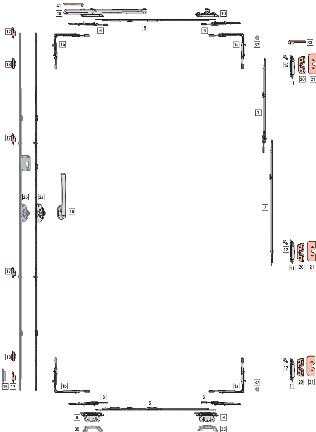
Илл. 3.1: на рис.: ПВХ, исполнение с левым открыванием согласно DIN; ШСФ 900 мм; ВСФ 1800 мм; запор DM 35
